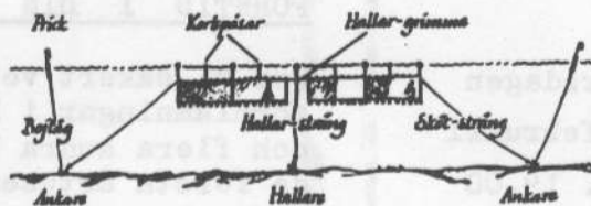
Sköt-lång med 4 skötar och en mitt-hallare (med 6 skötar 2 mitt-hallare)
